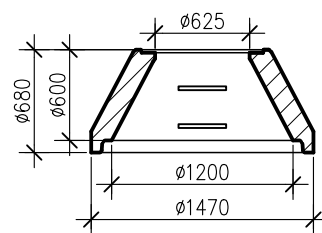
PRZEKRÓJ B-B
