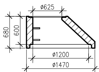
PRZEKRÓJ A-A
